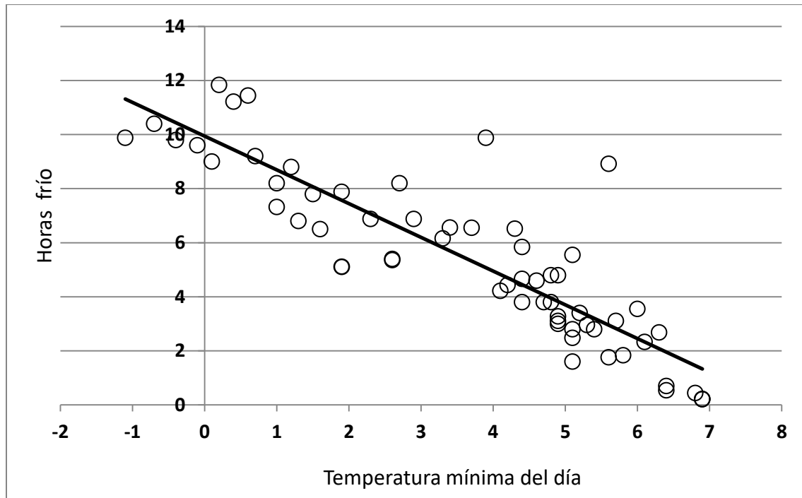
FIGURA 6. Gráfica de correlación entre las temperaturas mínimas y las horas frío.
