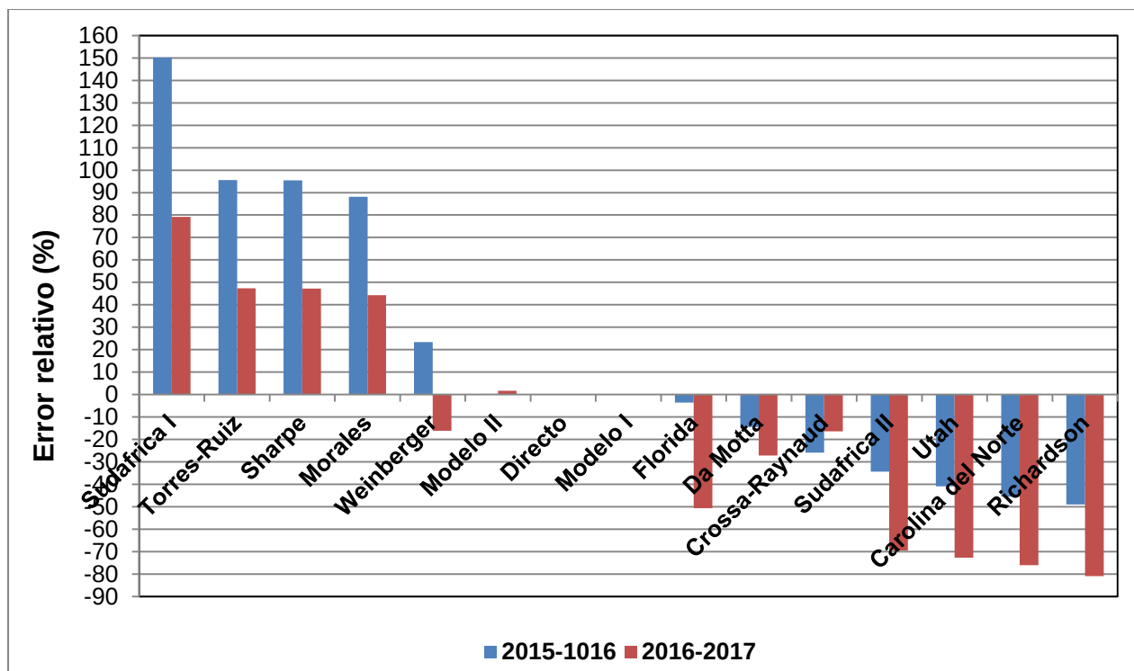
FIGURA 10. Error relativo porcentual de las horas frío calculadas por los métodos indirectos comparados con el registro del método directo en Chapingo, México (2015-2016 y 2016-2017).
