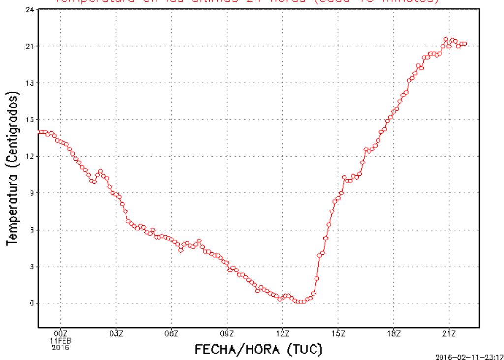
FIGURA 2. Gráfica de la marcha de la temperatura diaria.
